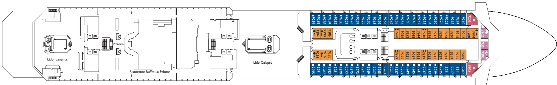
DECK 9 - AZZURRO
